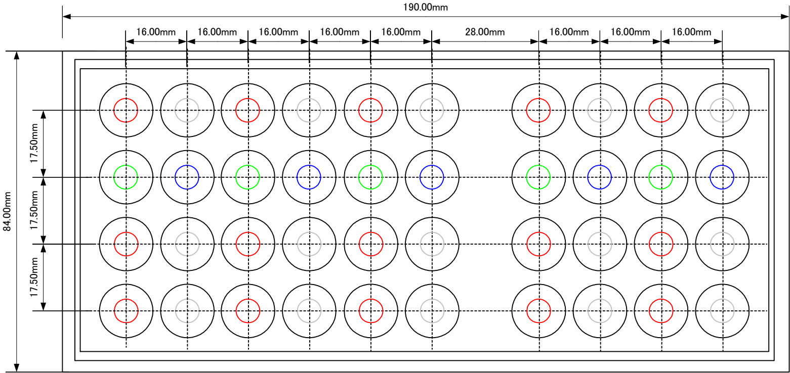
2x3系統 CH8-SEL2x3 WxHxD=190x84x200
